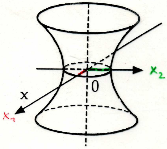
Einschaliges Hyperboloid
