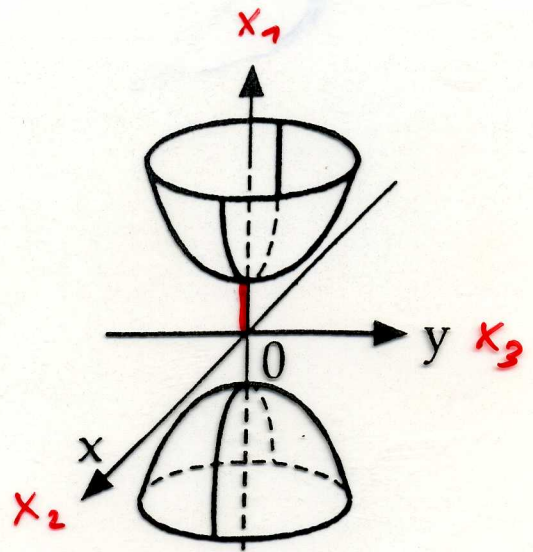
Zweischaliges Hyperboloid
