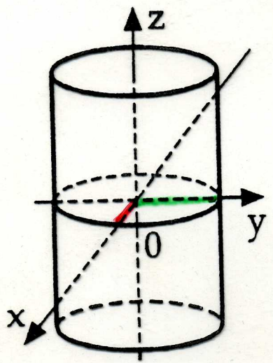
Elliptischer Zylinder
